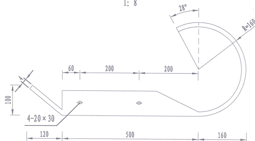
端头大样图
