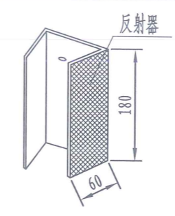
附着于砼护栏上的轮廓标侧面图
