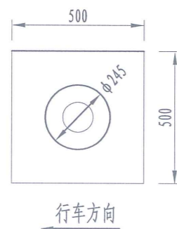
基础II平面图
