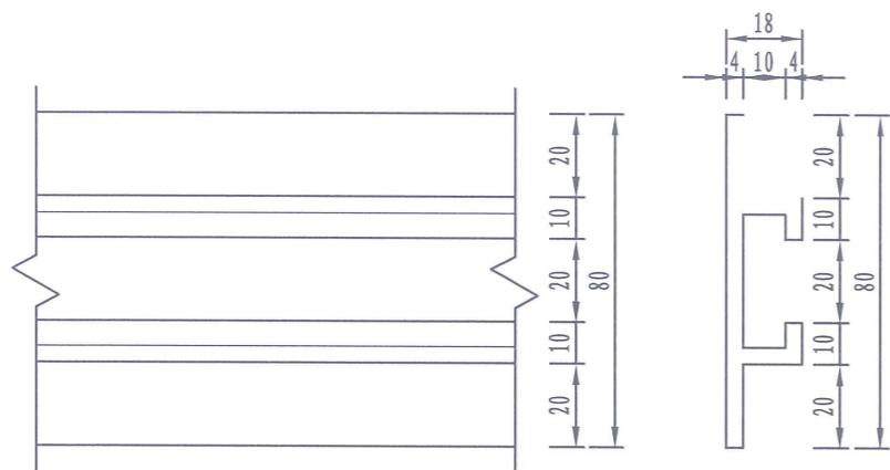
滑动槽钢 1:2
