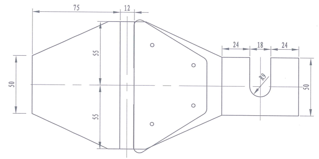
附着于砼护栏上的轮廓标正面图
