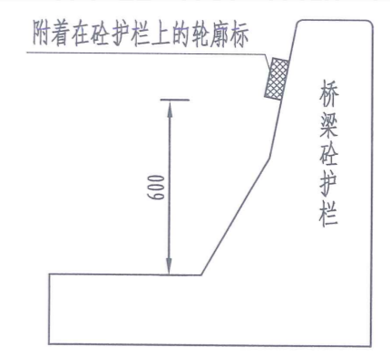
桥梁砼护栏轮廓标布设示意图
