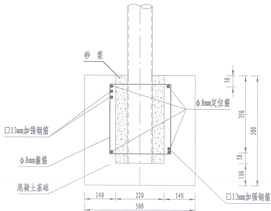
钢筋大样图
