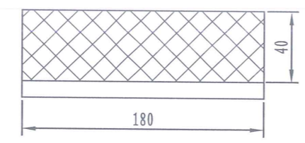
附着于砼护栏上的轮廓标正面图
