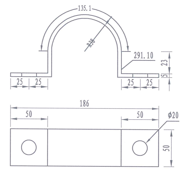
抱箍大样图 1:3
