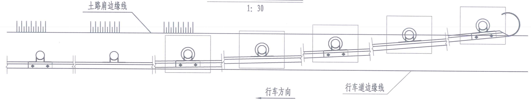
路侧护栏上游端部平面图
