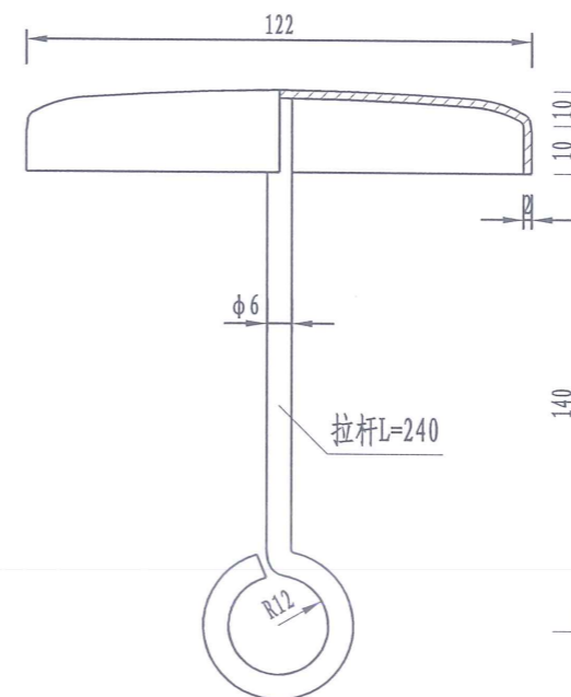
柱帽大样图
