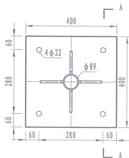
加劲法兰盘 1:10
