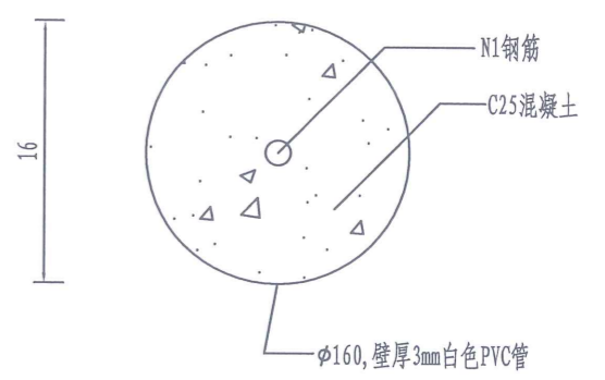
I-I 1:5
