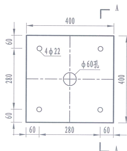
底座法兰盘 1:10
