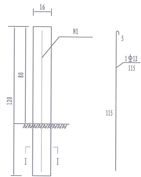
示警桩结构图 1:10
