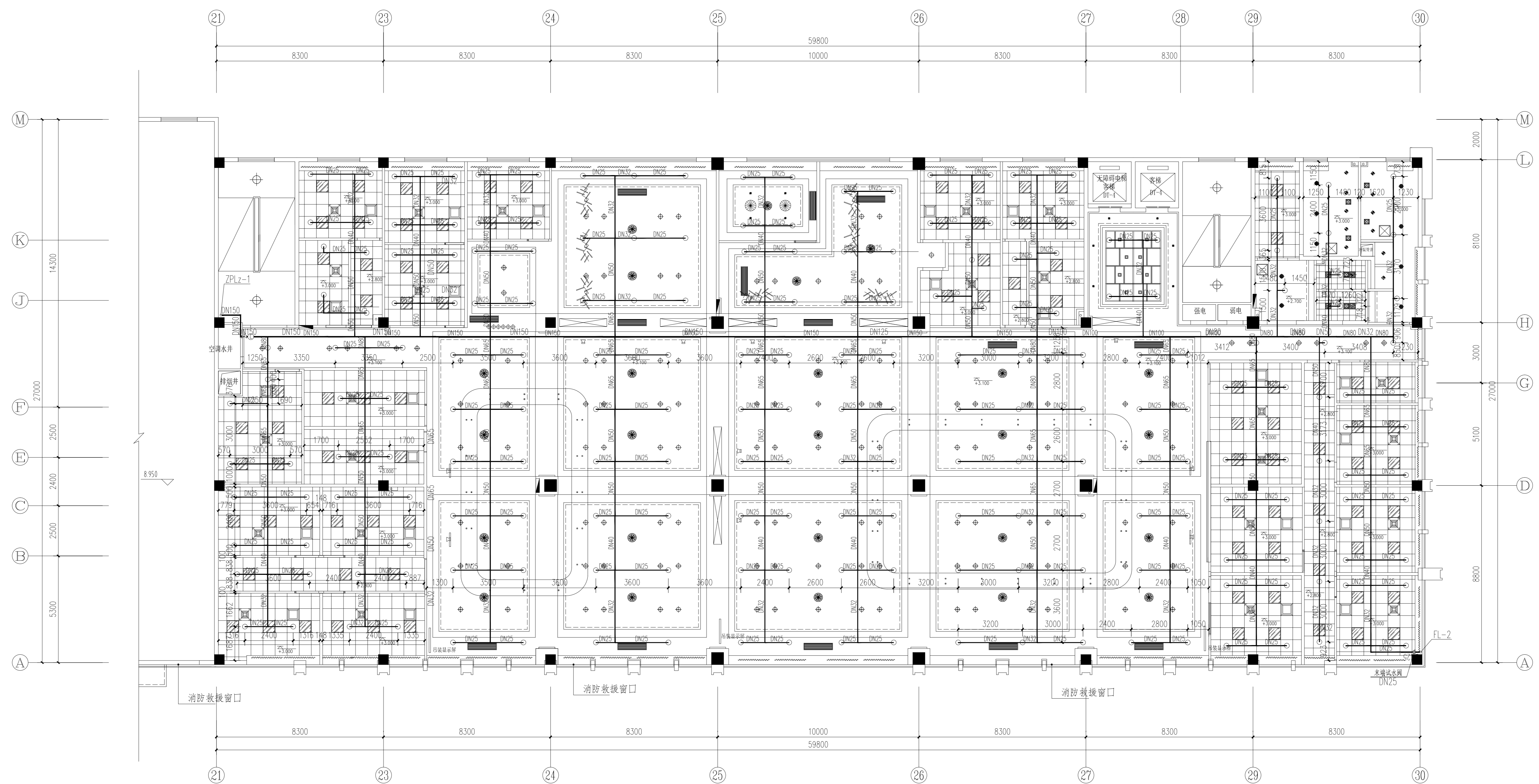
三层自动喷淋平面图 1:100
