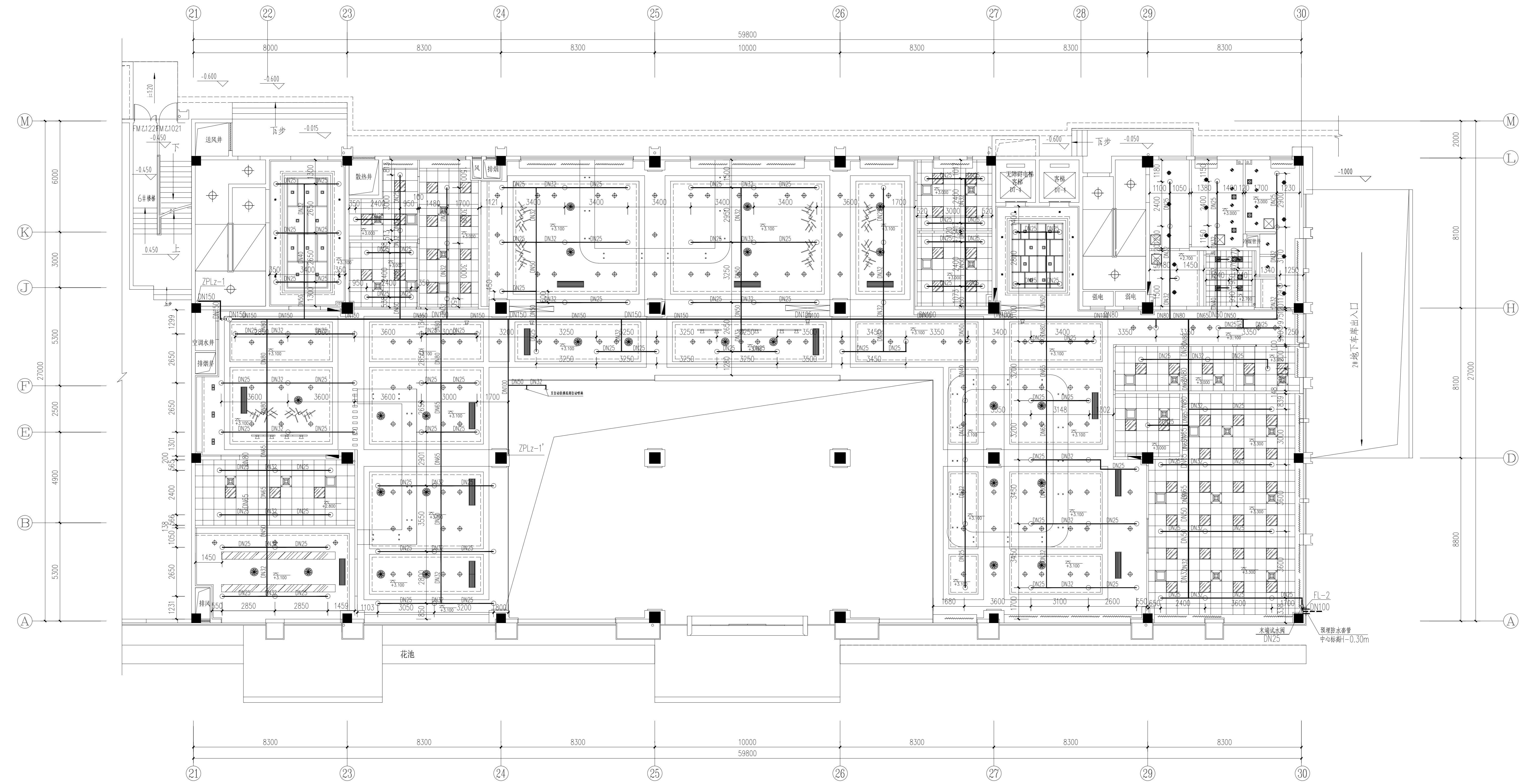
一层自动喷淋平面图 1:100
