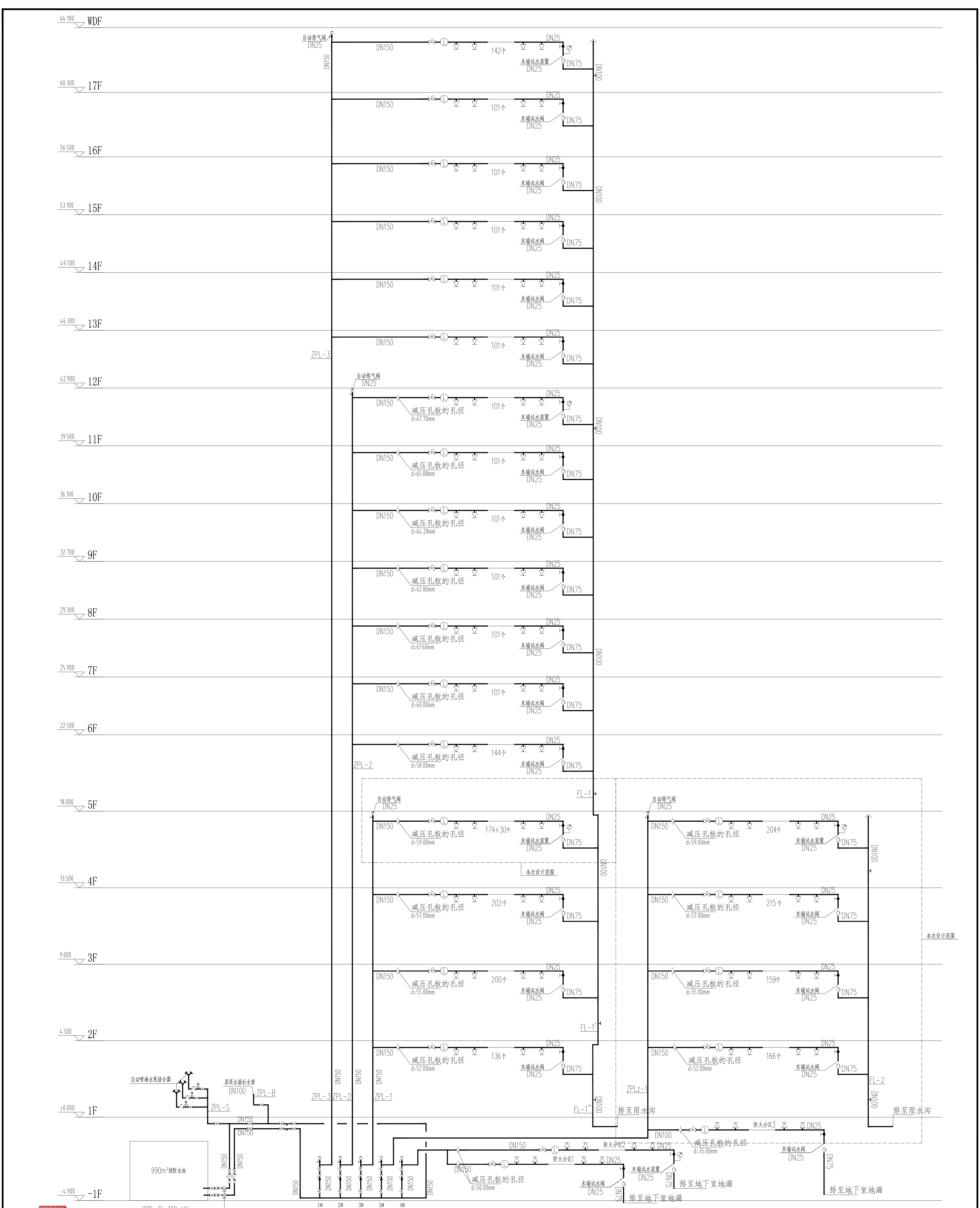
自动喷淋管道展开系统图
