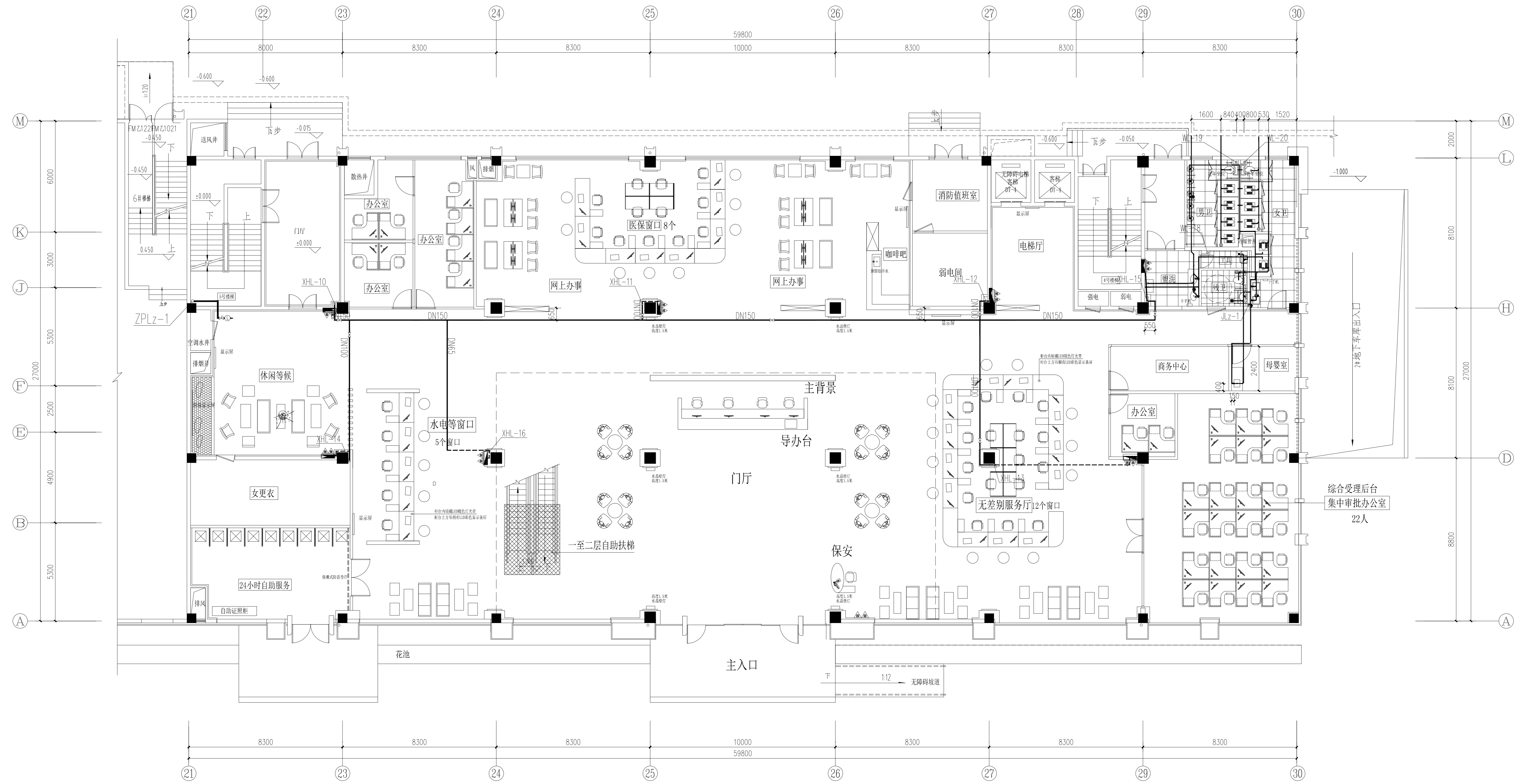
一层给排水平面图 1:100
